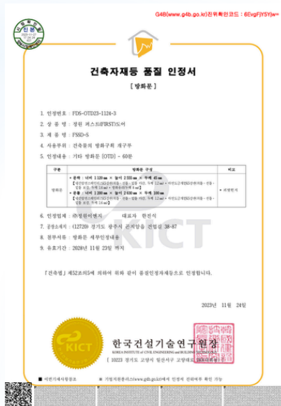
방화유리문 양개
