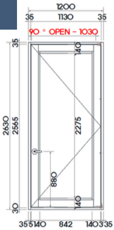
방화유리문 편개
