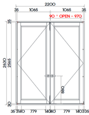
방화유리문 양개
